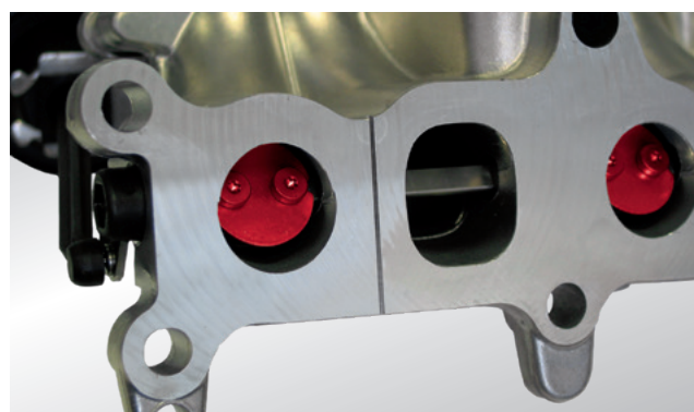
Fig. 2: Dois canais para cada cilindro: Válvulas de turbulência (destacadas a vermelho) no tubo de aspiração Pierburg, p. ex., no Opel Astra J 1.7 CDTi
